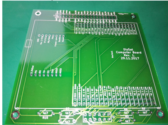
Tietokonelevy
