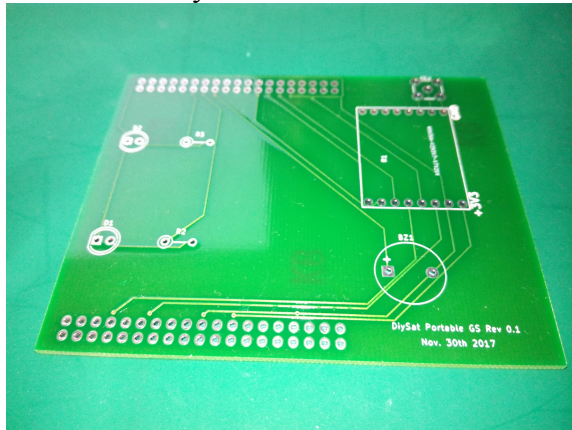
Maa-asemalevy
