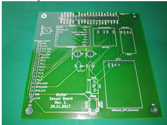
Anturilevy
